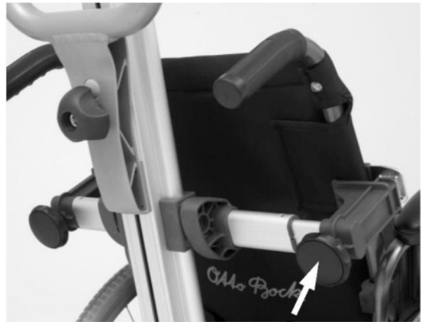
Утримуючий затискач
